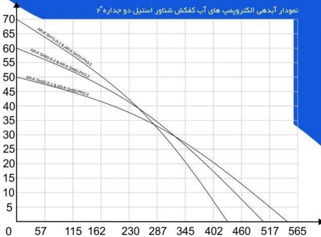
جدول آبدهی الکتروپمپ های کفکش شناور استیل تک فاز و سه فاز دو جداره ۲"
